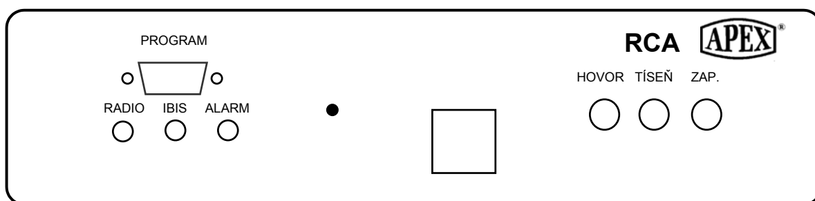
Obr.1. Přední panel radiokomunikačního adaptéru RCA 06
